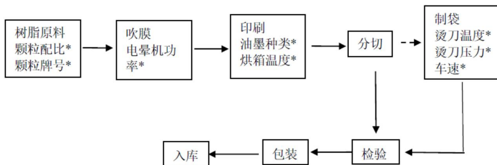
图3-9 PE膜制袋产品
