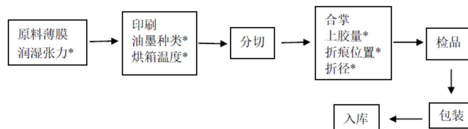
图3-4 标瓶产品工艺流程图
