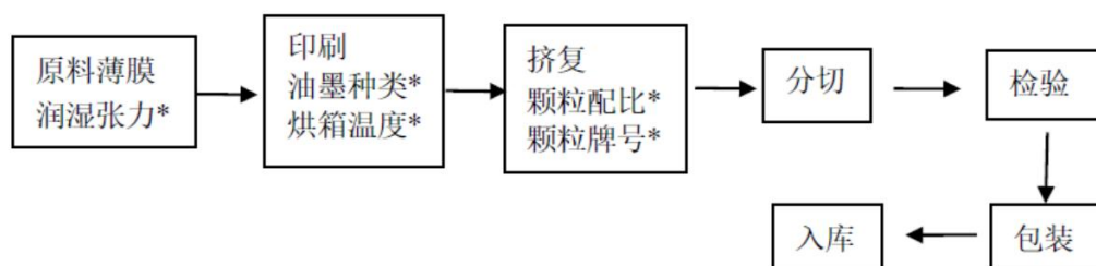
图3-3 挤复产品工艺流程图
