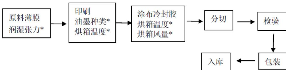
图3-7 冷封胶表印产品
