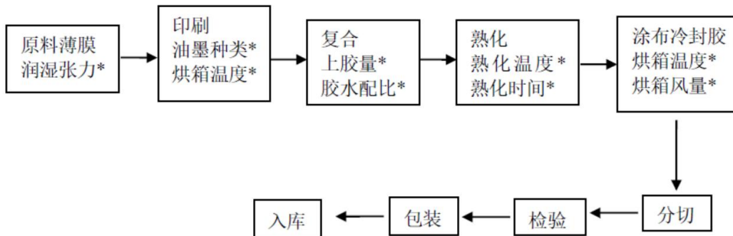
图3-8 冷封胶复合产品
