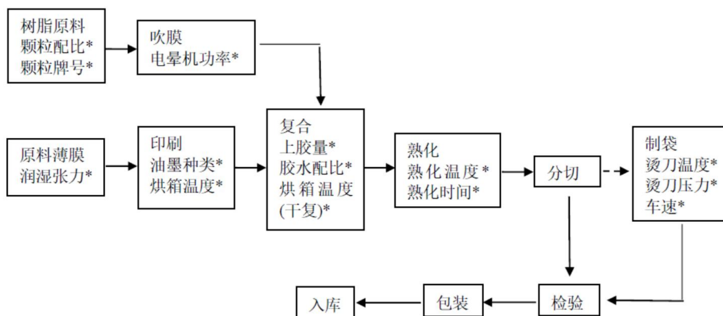
图3-2干复（无溶剂）产品工艺流程图
